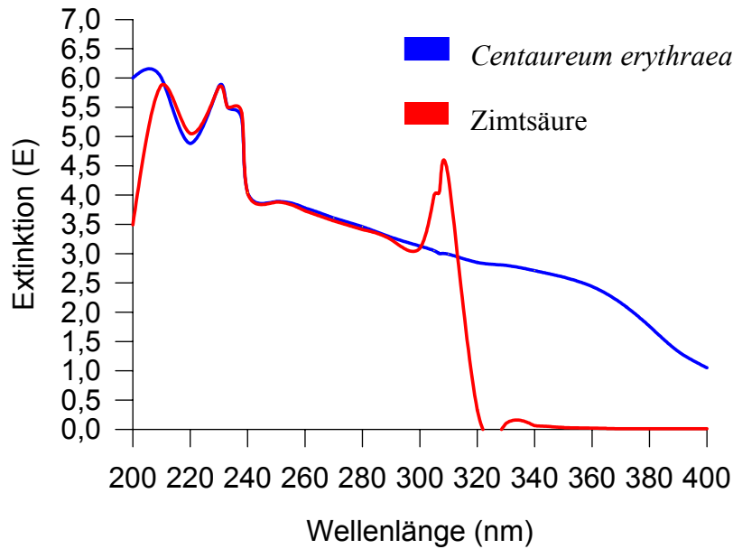
Abb. 14: Absorptionskurve von Zimtsäure (0,5 % in H 2 O) und Centaureum erythraea (1,2 %, 1:1 verdünnt) im Wellenlängenbereich von 200-400 nm.
